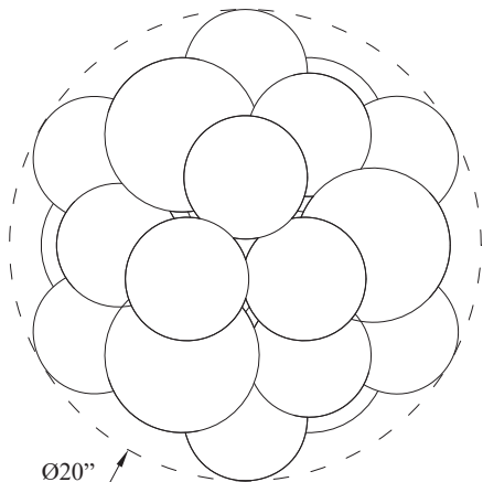
Top view Vue de dessus
