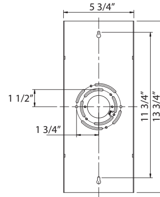
WS-W37916 & WS-W37922 Backplate
