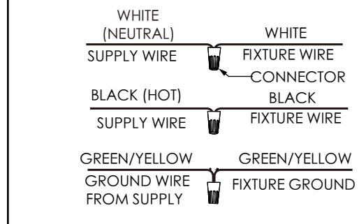
Fig. 4 Wiring guide
