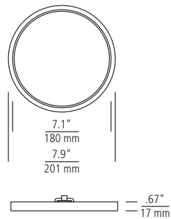
TRAVERSE LOTUS ROUND 7" 14927RD-15
