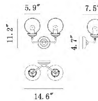
DU95 E26×2 Max60W
