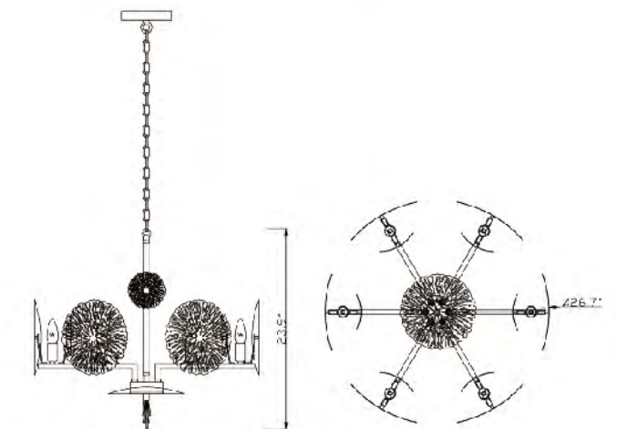
ZL19 E12×6 Max40W
